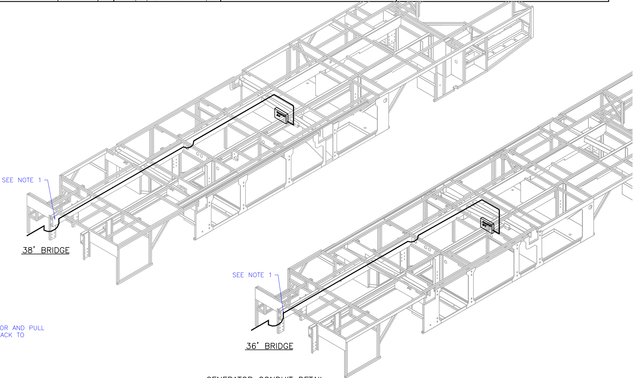
GENERATOR CONDUIT DETAIL
